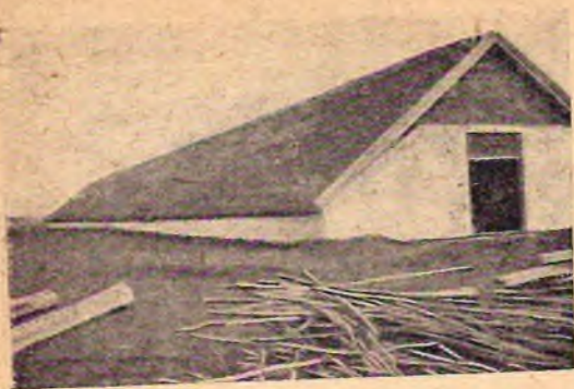
Кошара типа 1931 г. Вид с севера
