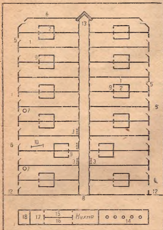
СХЕМАТИЧ. ПЛАН СВИНАРНИКА
